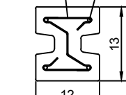
DETALHE 1 - SEÇÃO DA COLUNA E FERRAGEM
